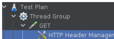
Рисунок 3 – Добавление менеджера заголовков к запросу GET
