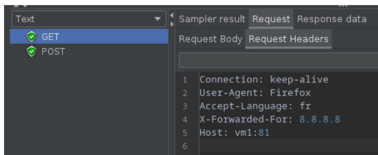
Рисунок 6 – Результат подмены заголовка
