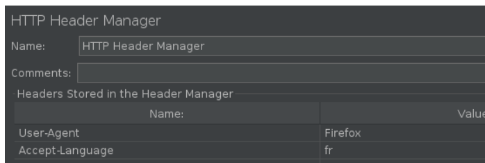
Рисунок 4 – Уникальные заголовки для GET-запроса
