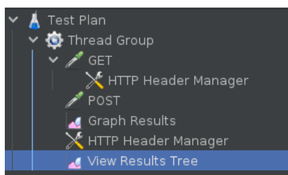
Рисунок 5 – Добавление слушателя результатов
